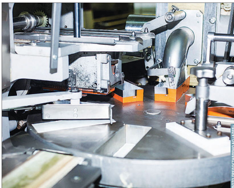
Линия по производству сливочного масла
